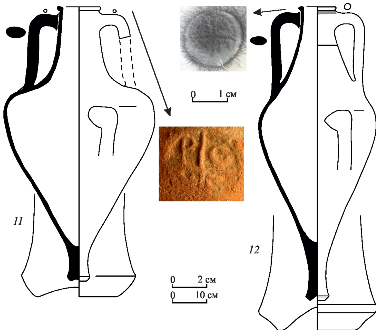
Рис. 3. 11 — амфора типа II из погребения № 412 Прикубанского некрополя; 12 — амфора варианта III-A из кургана у с. Богачевка.
