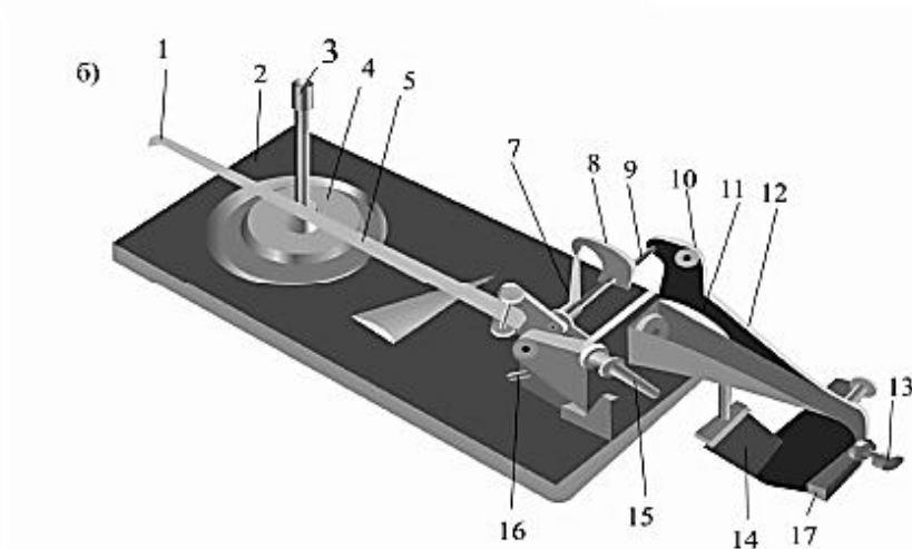
Рисунок 3.5 - Термограф метеорологический
