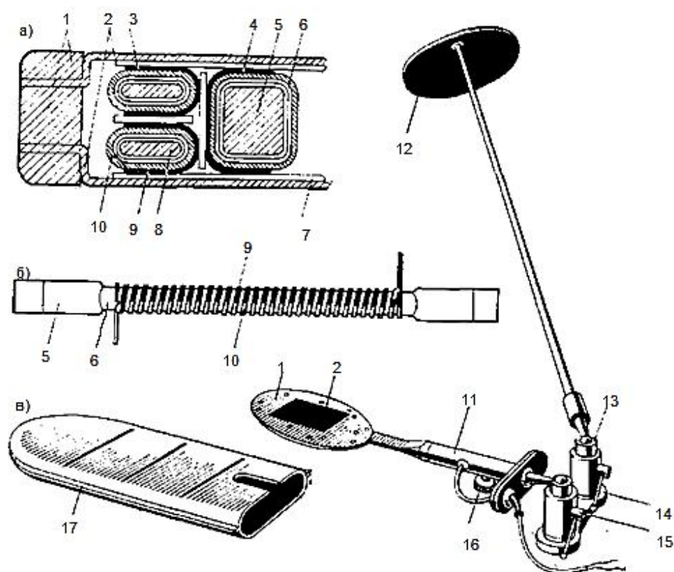
Рисунок 9.6 - Балансомер М-10М
