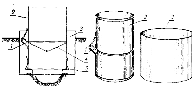
Рисунок 7.2 - Почвенный дождемер ГР-28
