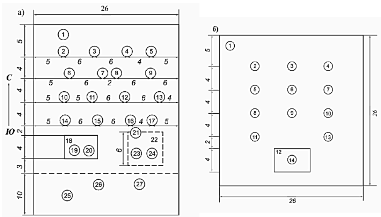
Рисунок 2.1 - План размещения оборудования и приборов на метеорологической площадке (расстояния указаны в метрах):
