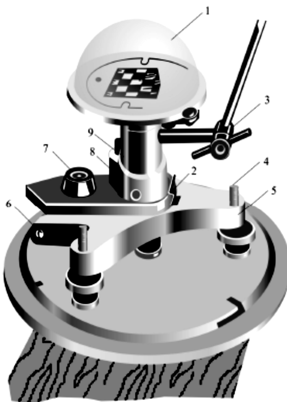
Рисунок 9.4 - Термоэлектрический пиранометр М-80М
