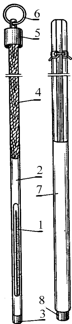
Рисунок 3.9 – Устройство вытяжного термометра
