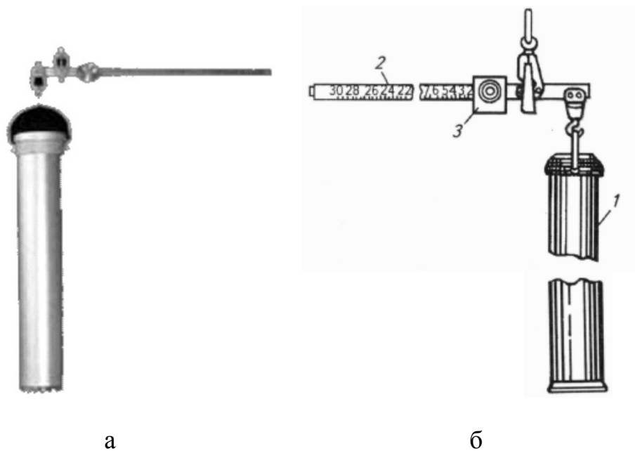
Рисунок 7.6 - Снегомер весовой ВС-4
