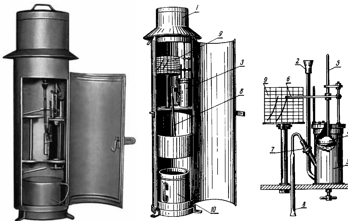
Рисунок 7.3 - Плювиограф П-2
