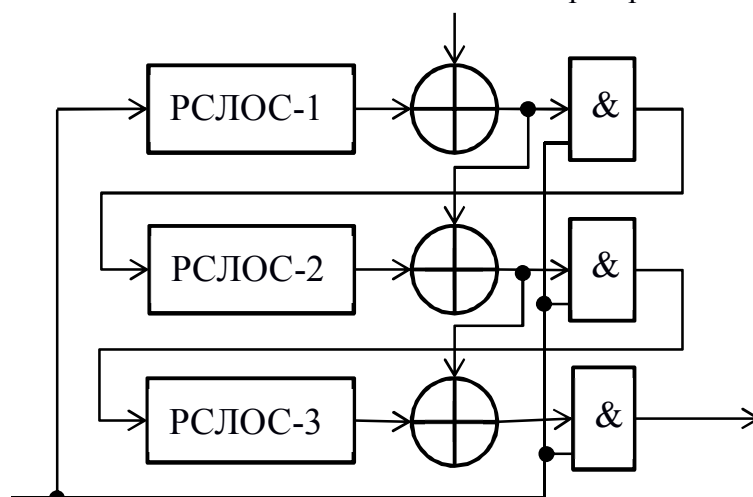
Рисунок 3.8. Схема генератора Голлмана.
