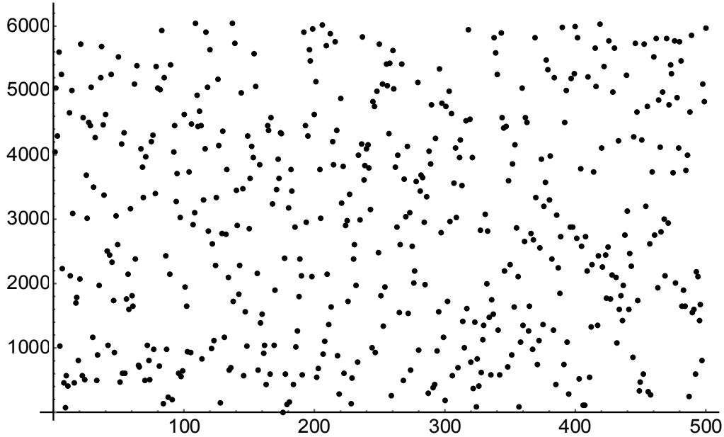
Рисунок 3.1. График ЛКП для X_0 = 7, a = 106, c = 1283, m = 6075 .
