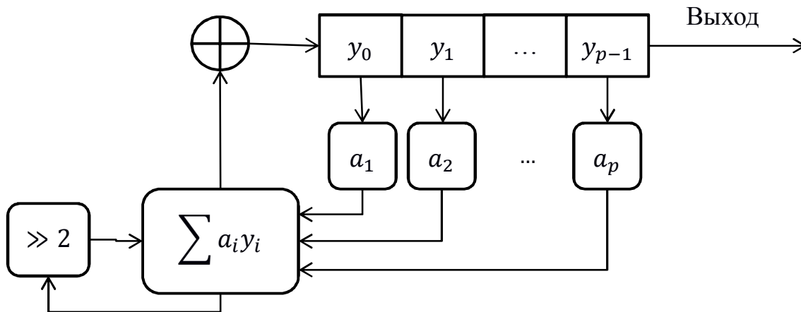
Рисунок 3.6. Схема PCOSP.
