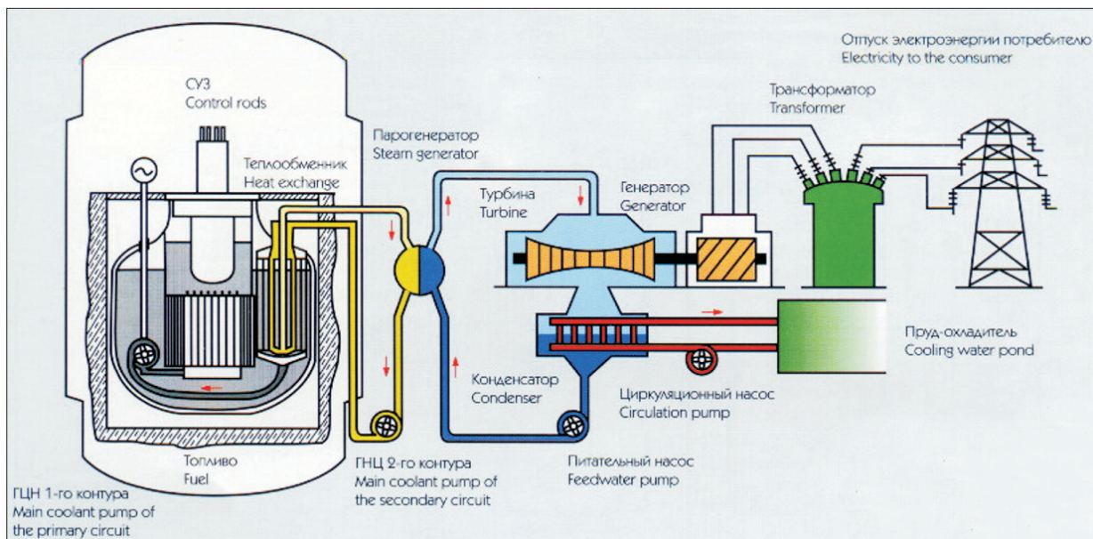
БН-600 – реактор на быстрых нейтронах. Автор проекта – академик Ф.М. Митенков
